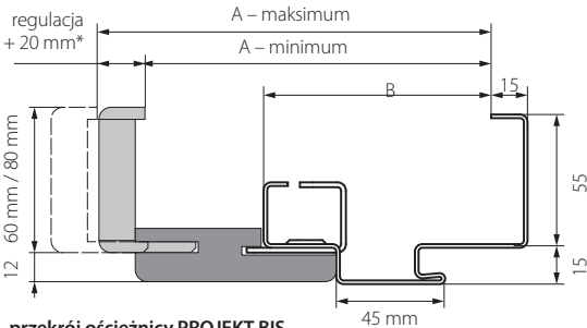
przekrój ościeżnicy PROJEKT BIS * dla zakresu A regulacja +15 mm
