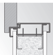
ościeżnica Kątowa DUŻA montaż na ścianie kartonowo-gipsowej
