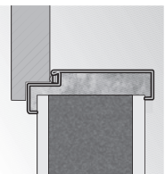
montaż bez dodatkowych elementów kotwiących
